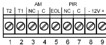
Fig. 5 Terminal block I Bloque de terminals I Plaque à bornes I Morsettera I Opis zacisków
