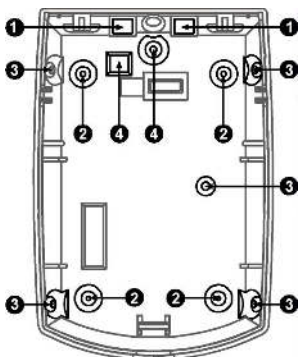
Fig 2 Knockout holes | Orificios troquelados | Trous de débouchure | Fori ciechi | Otwory montażowe
